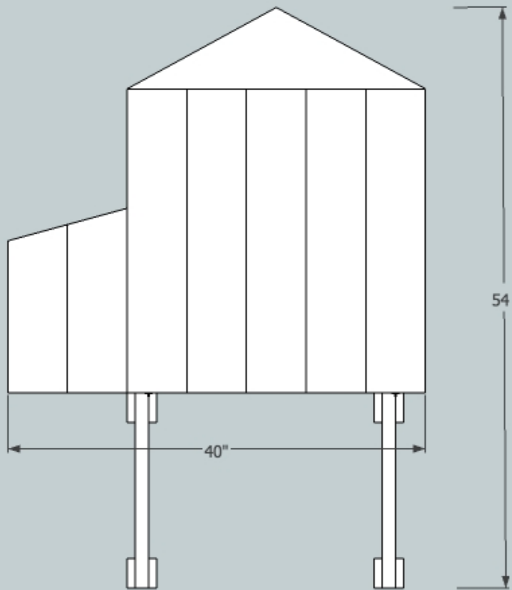
Cottage Face Dimensions
